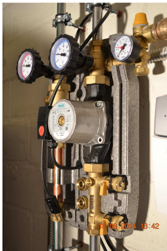
Solarstation mit Thermo-, Flow- und Manometer u. Überdruckventil
